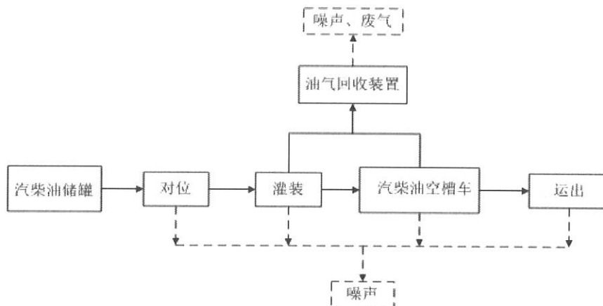
图3 汽柴油、化工产品装车工艺流程及产污环节图
